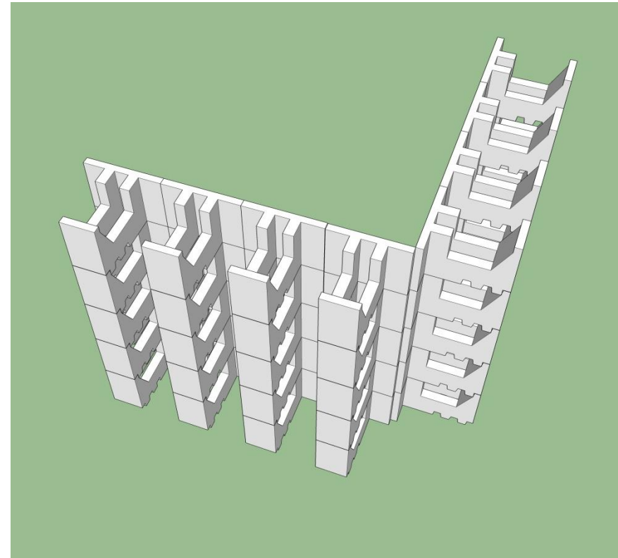
Mur avec angle droit intérieur
