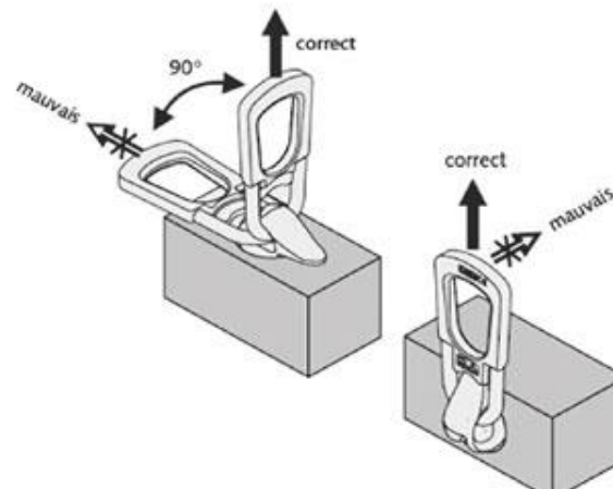
2. Levage
