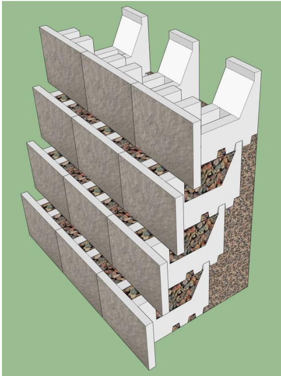
Mur avec un fruit
